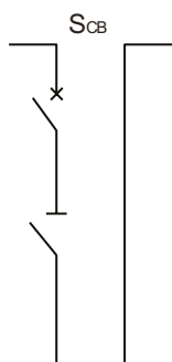
Ячейка секционирования с силовым выключателем
